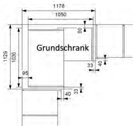
90° Ecke, 2-türig
